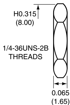
NUT
